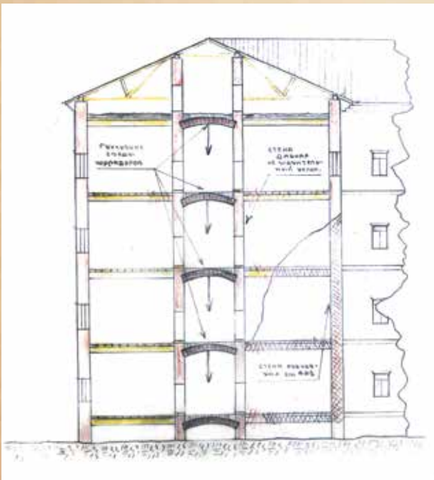
Разрез здания на Обводном канале, 19
